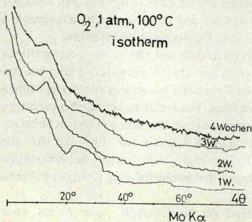
Fig. 10. Densitometerkurven der Molybdän-Röntgendiagramme von Produkten eines isothermen Zersetzungsversuchs, \text{O}_2 -Atmosphäre, 100^\circ\text{C} .
